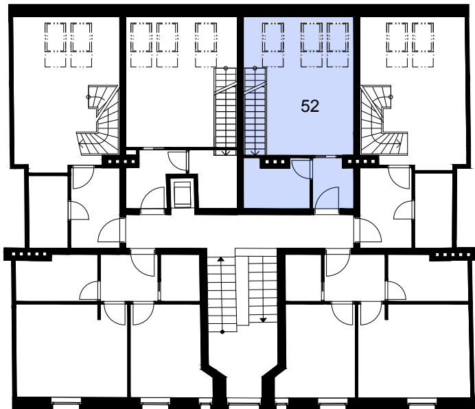
SCHÉMATICKÝ PŮDORYS
