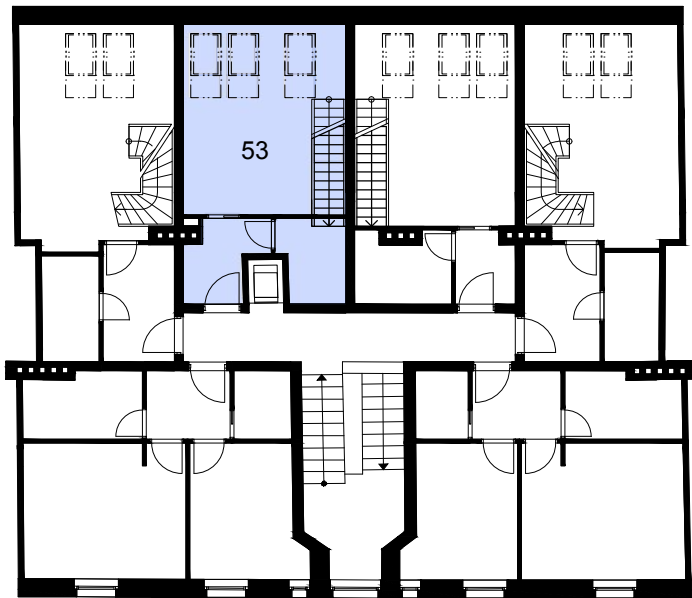
SCHÉMATICKÝ PŮDORYS
