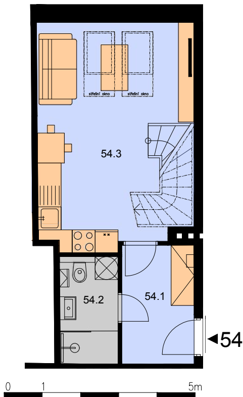
SCHÉMATICKÝ PŮDORYS
