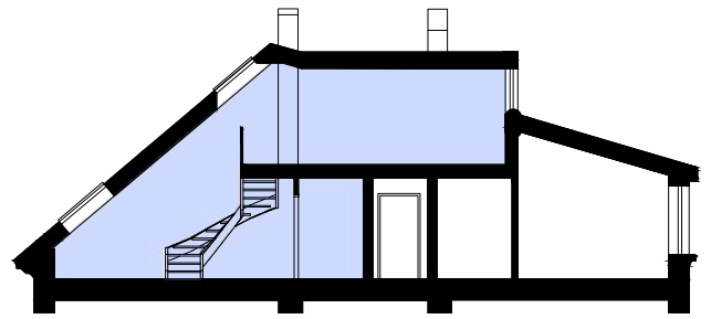
SCHÉMATICKÝ ŘEZ
